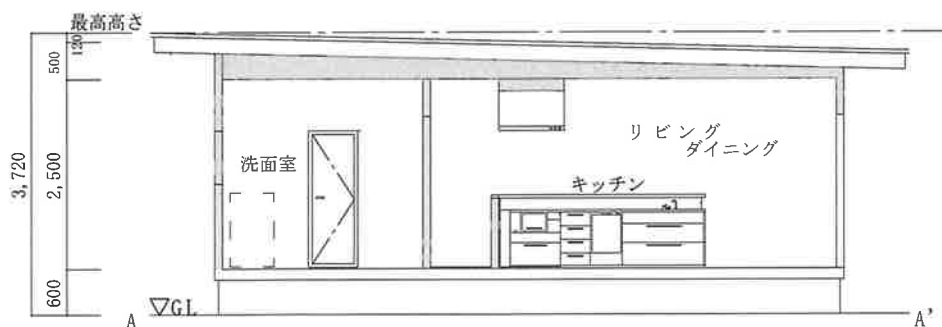
断面図
