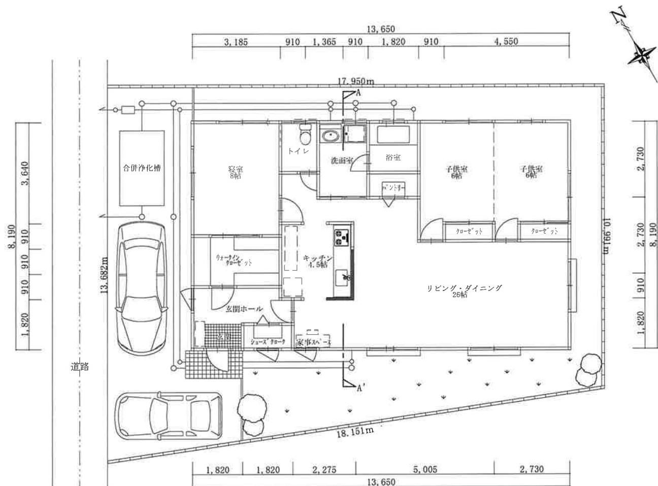
平面配置図
