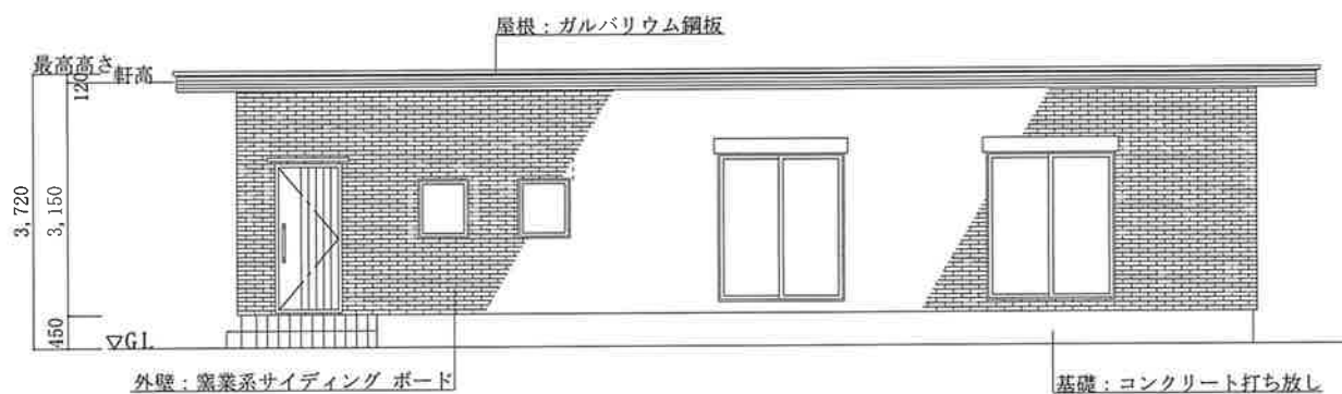
南側立面図
