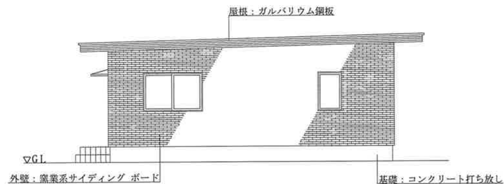
西側立面図
