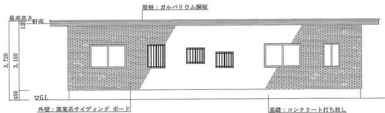
北側立面図
